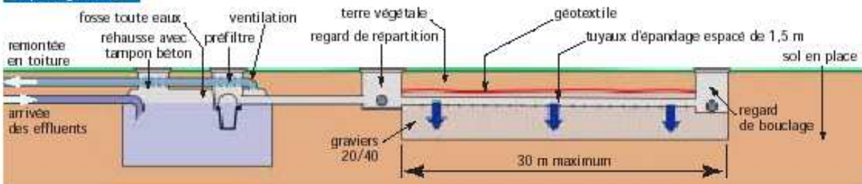
Coupe longitudinale
