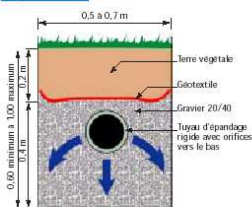
Coupe transversale
